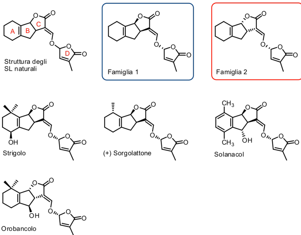
Figura 2. Struttura chimica dei principali strigolattoni naturali.
