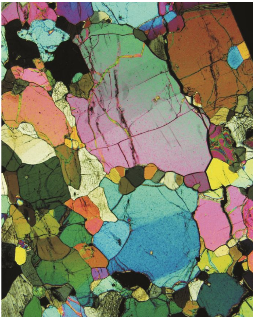
Fig. 1 - Roccia di mantello (peridotite) al microscopio ottico polarizzato. 10 ingrandimenti
