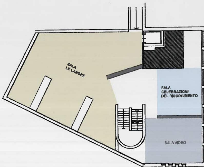
PIANO PRIMO
